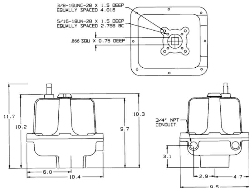
CL Dimensions
