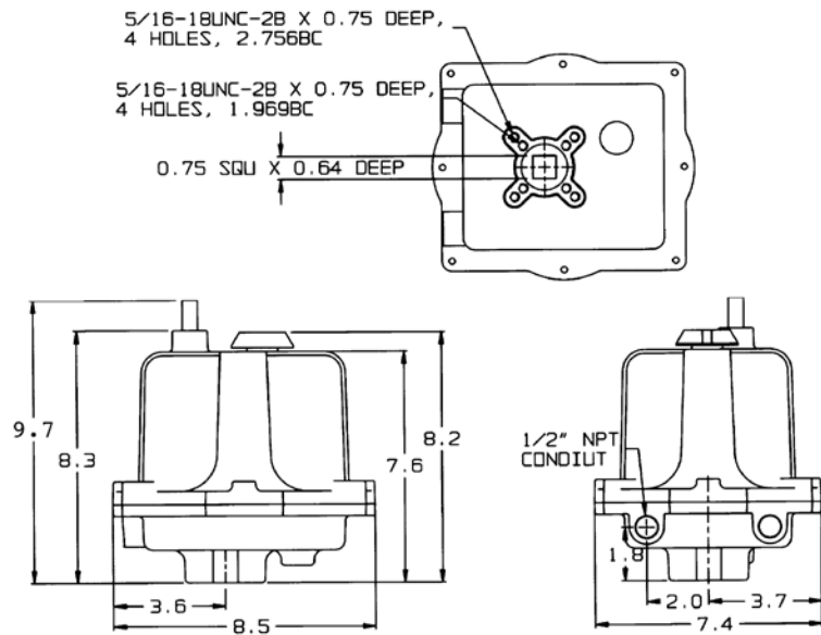
CS Dimensions
