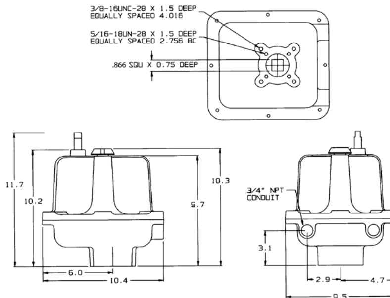
CL Dimensions
